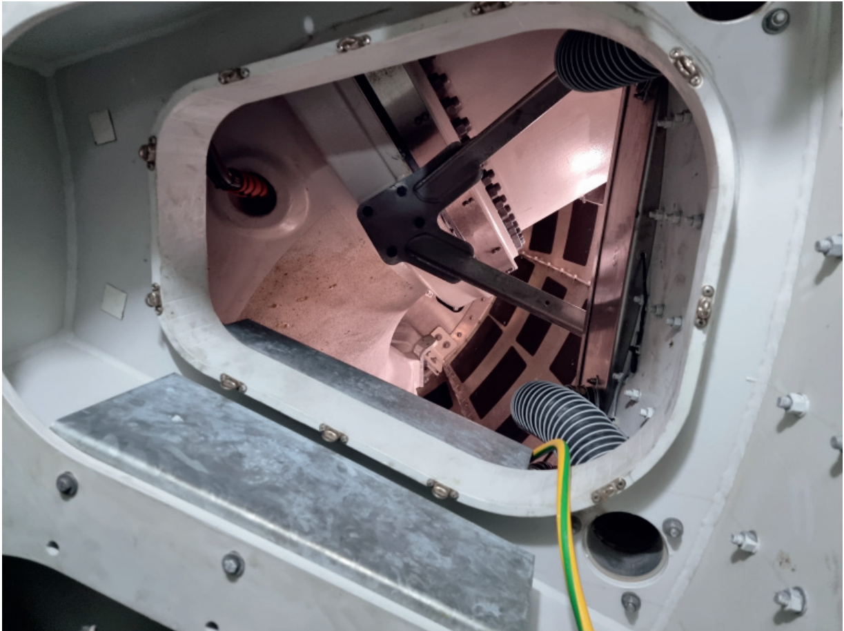
Dalby december 2021, passage ut till navet med infästning av blad synligt
